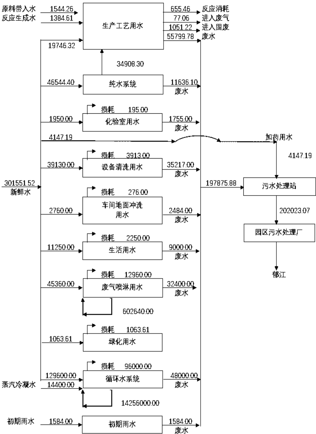
图 2.4.10-1 项目水平衡单位：m³/a
