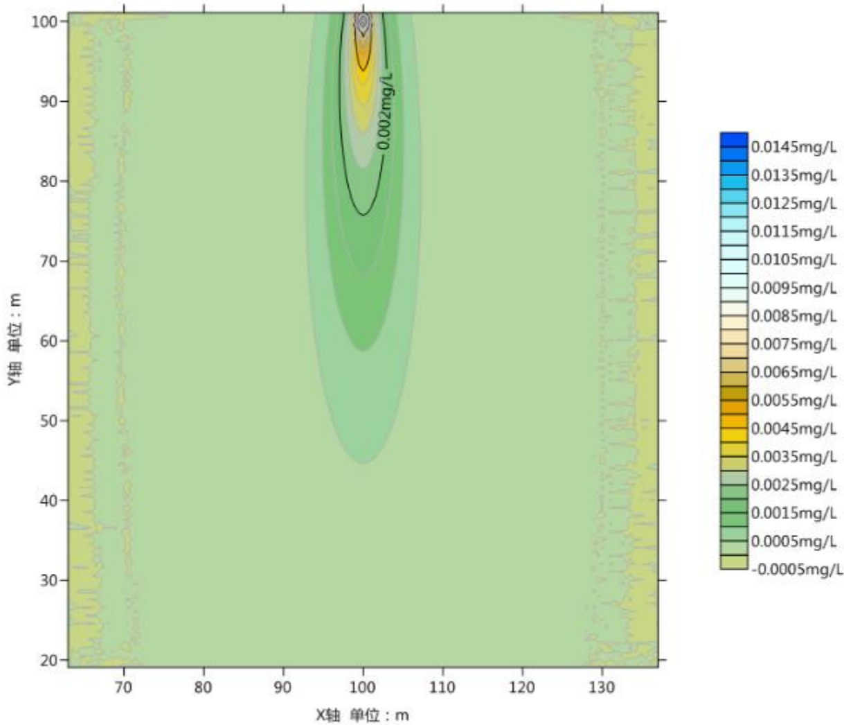
图 4.2-29 连续泄漏第 100 天，污水处理站二氯甲烷污染扩散范围图
