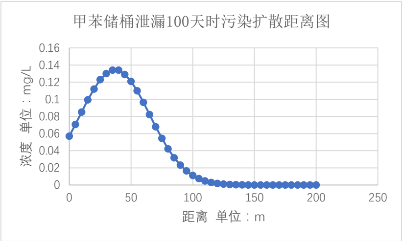
图4.2-25 甲苯储桶泄漏100天，甲苯污染扩散距离图
