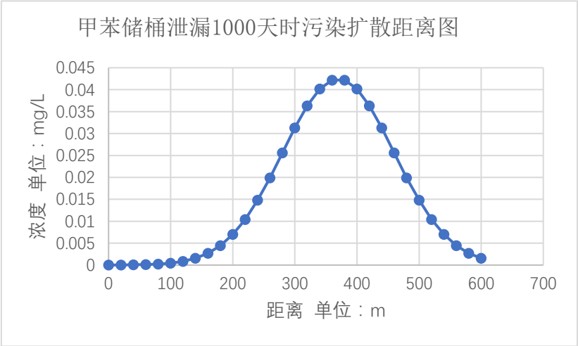
图4.2-26 甲苯储桶泄漏1000天，甲苯污染扩散距离图
