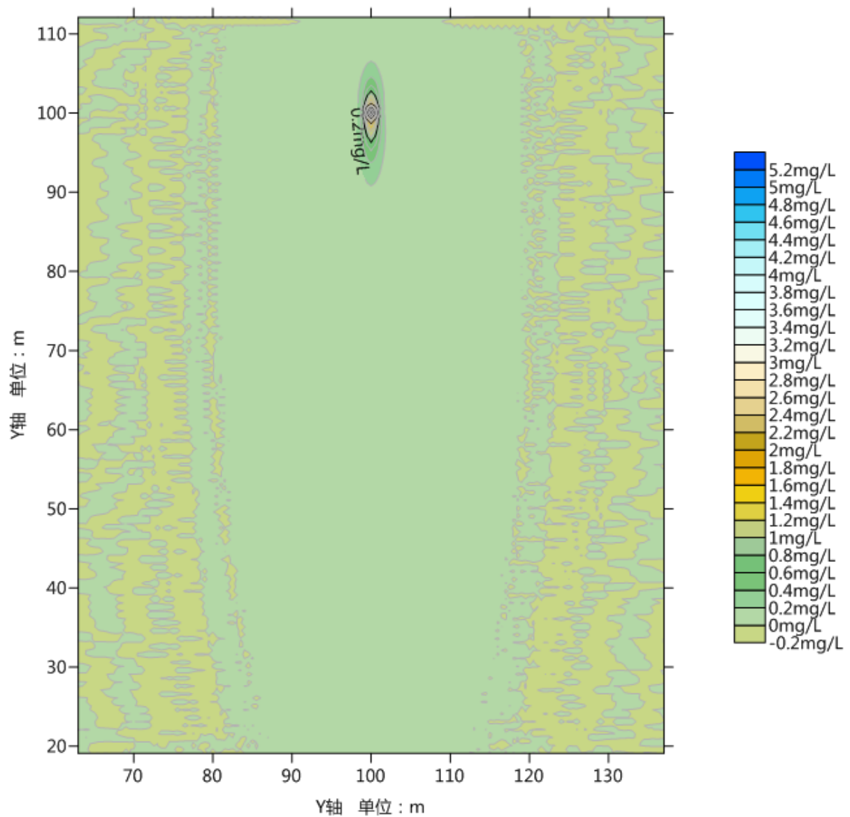
图4.2-27 连续泄漏第100天，污水处理间COD污染扩散范围图
