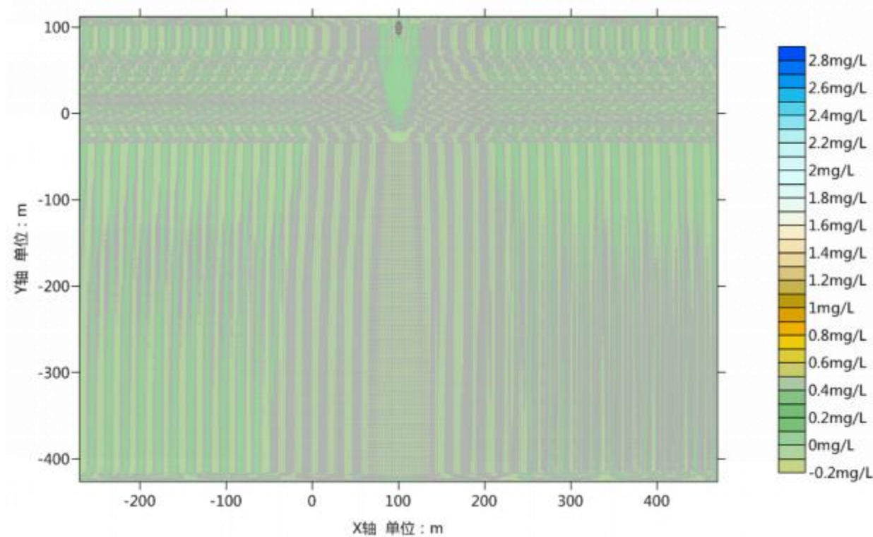
图 4.2-28 连续泄漏第 1000 天，污水处理间 COD 污染扩散范围图
