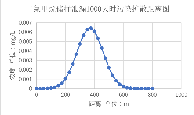
图4.2-24 二氯甲烷储桶泄漏1000天，二氯甲烷污染扩散距离图
