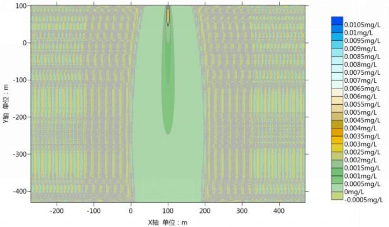
图 4.2-30 连续泄漏第 1000 天，污水处理站二氯甲烷污染扩散范围图
