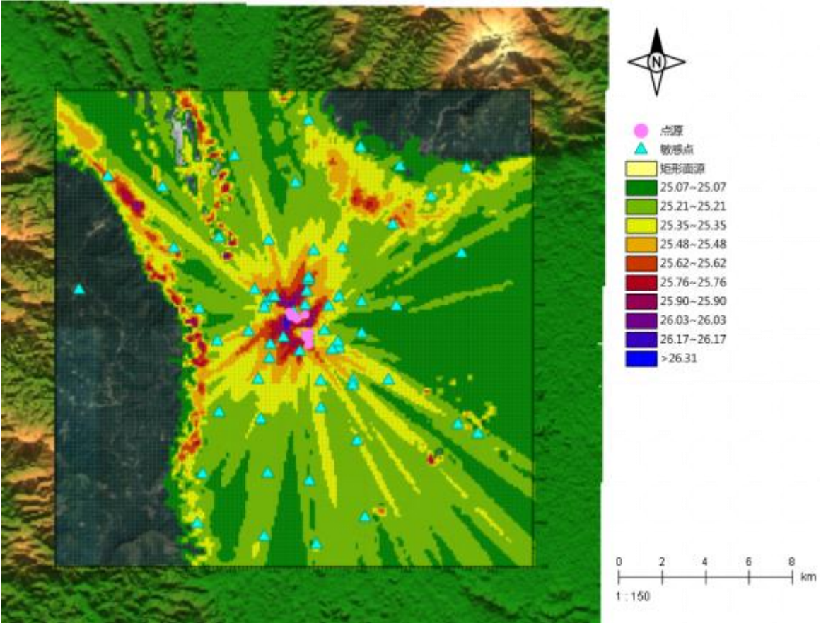
图 4.2-11 正常排放条件下甲醇日平均浓度等级线图（预测值）
