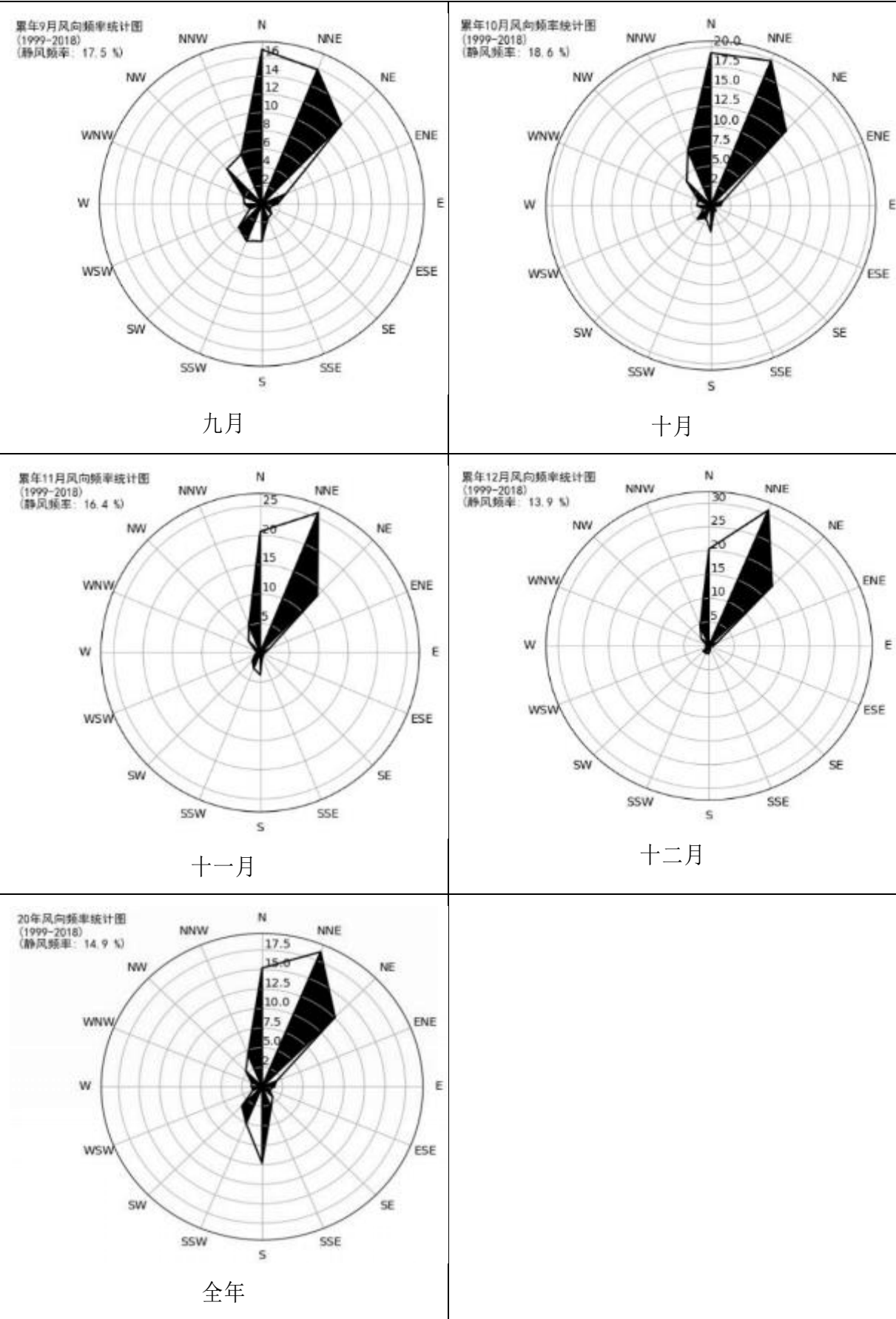
图 4.2-1 横县月和风向玫瑰图 (1999-2018 年)
