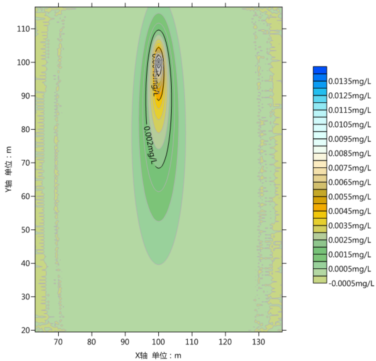
图 4.2-31 连续泄漏第 100 天，污水处理站甲苯污染扩散范围图
