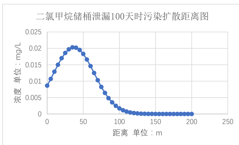
图4.2-23 二氯甲烷储罐泄漏100天，二氯甲烷污染扩散距离图
