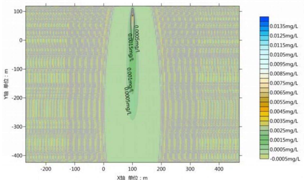
图 4.2-32 连续泄漏第 1000 天，污水处理站甲苯污染扩散范围图
