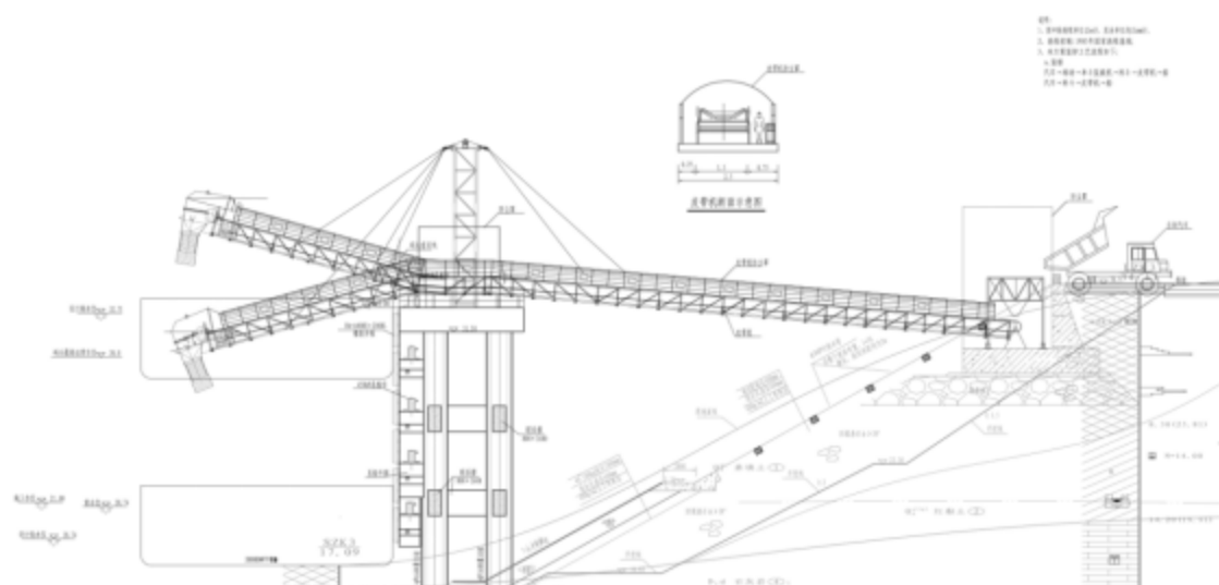
图 2.3-1 装卸工艺示意图
