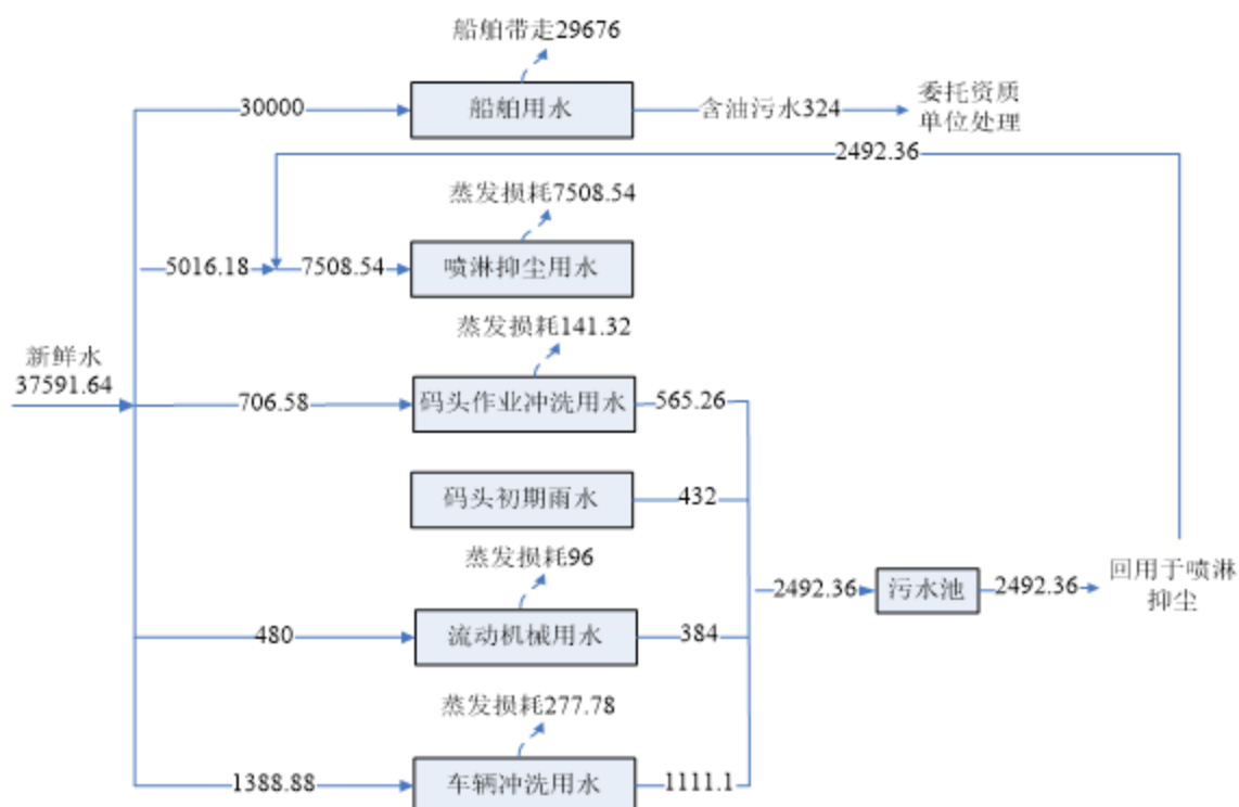
图 2.3-1 本工程水平衡图单位: \text{m}^3/\text{a}
